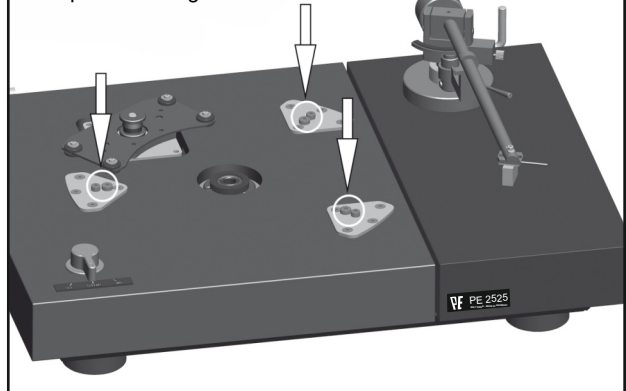
F 1 - Lösen und Entfernen der Transportsicherungsschrauben
